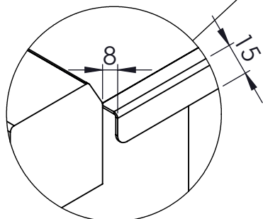
DETTAGLIO SCALA 1 : 2
